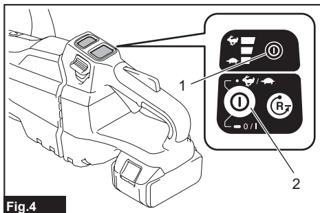
Fig.4 ► 1. Témoin d'alimentation 2. Bouton d'alimentation principale
